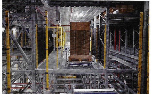
Hörmann Logistik lieferte die gesamte Fördertechnik zur Anbindung des neuen Hochregallagers und für die Versandbereitstellung.
