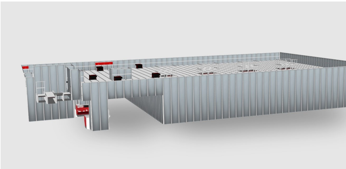
Abbildung 1 Visualisierung des AutoStoresystems mit Kommissioniertunnel
